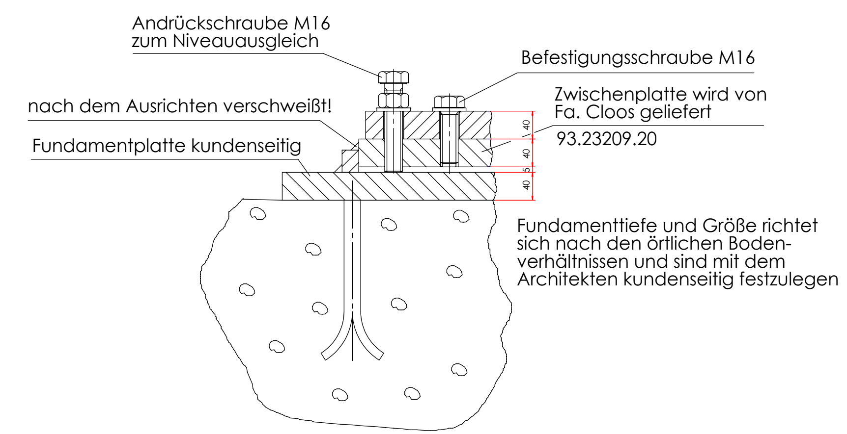
Befestigungsprinzip: C-Ständer programmierbar M 1:5
